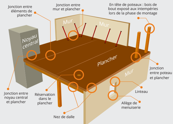
Représentation des points singuliers pouvant potentiellement retenir l'eau en phase chantier
