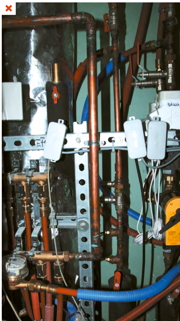
Absence d'isolation des tuyaux de chauffage et d'eau chaude sanitaire du module thermique d'appartement dans la gaine technique. ©AQQC
