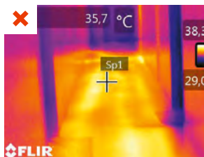
Bouclage d'eau chaude sanitaire noyé dans la dalle sans isolation.
