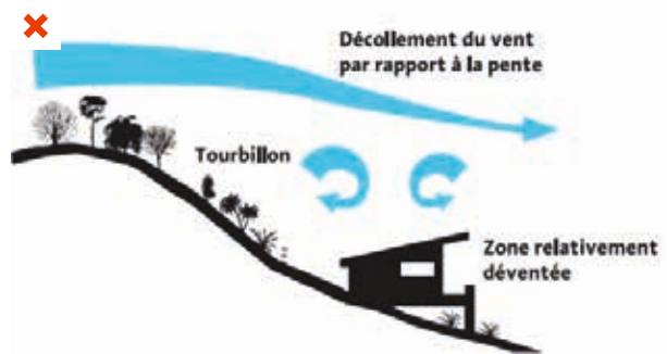
Site sous le vent des collines ou de dénivelés. L'effet de décollement provoque des vents contraires et crée une zone déventée défavorable à la ventilation naturelle. ©Guide Ecodom
