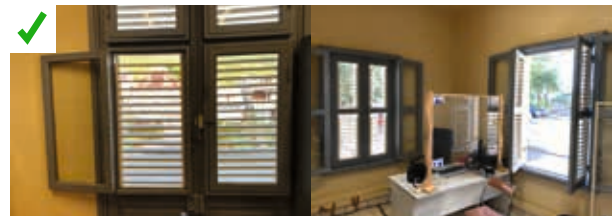
Menuiseries en bois disposant de ventelles réglables et de survitrages ouvrables individuellement. ©AQC
