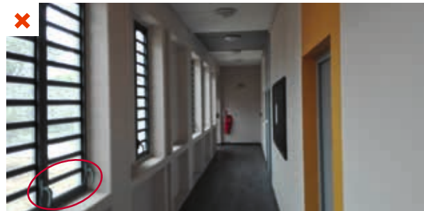
Jalousies réglables donnant sur un espace de circulation ne permettant pas de garantir un taux d'ouverture constant de 50 % de la façade. ©AQC
