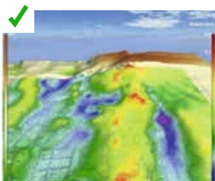
Exemple de visuel d'un logiciel permettant d'appréhender la vitesse du vent au regard de la topographie du site. ©MétéoDyn
