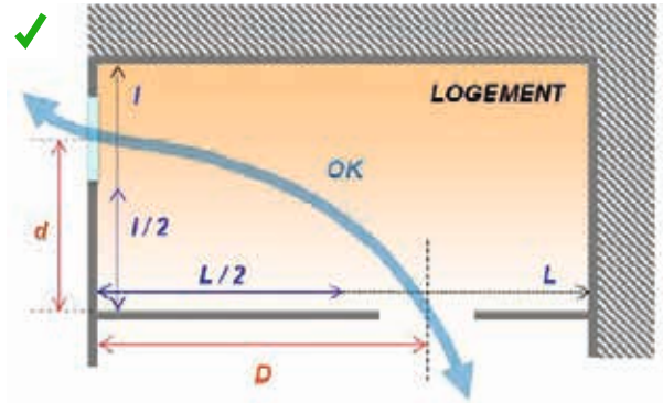
Schéma indiquant la distance minimale à respecter entre les ouvertures positionnées sur des façades adjacentes. ©RTAADOM
