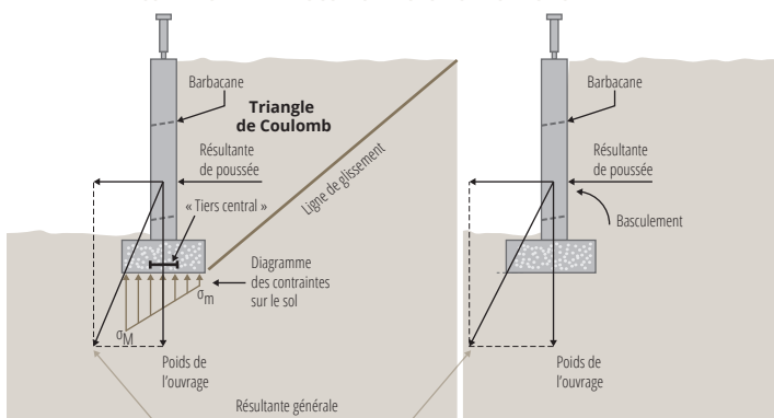
SCHÉMA SIMPLIFIÉ DES SOLlicitATIONS D'UN MUR-POIDS
