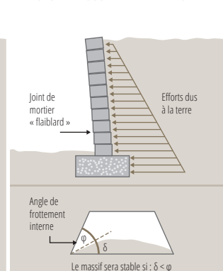
CAS DE BASCULEMENT DE PAROI
