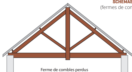
SCHEMAS DE SYSTEMES TRIANGULES (fermes de combles perdus ou aménageables)
