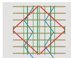
En rouge : les barres venant s'opposer au flambement des arbalétriers, appelées aussi « antiflambage ». En bleu : les barres dites de contreventement apportant à la charpente sa stabilité d'ensemble. En vert : des barres rejoignant les nœuds, ou barres filantes, appelées aussi « lisses sur entrait ».
