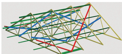
En rouge : les barres venant s'opposer au flambement des arbalétriers, appelées aussi « antiflambage ». En bleu : les barres dites de contreventement apportant à la charpente sa stabilité d'ensemble. En vert : des barres rejoignant les nœuds, ou barres filantes, appelées aussi « lisses sur entrait ».
